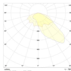
Asimétrico Frontal
