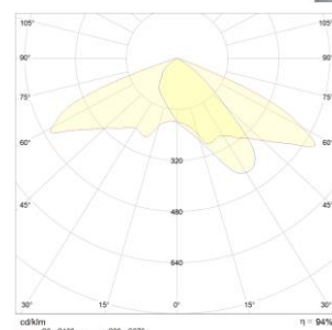
Asimétrico Longitudinal
